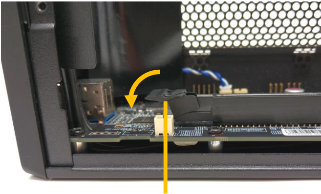
PCI Express スロットのロック
