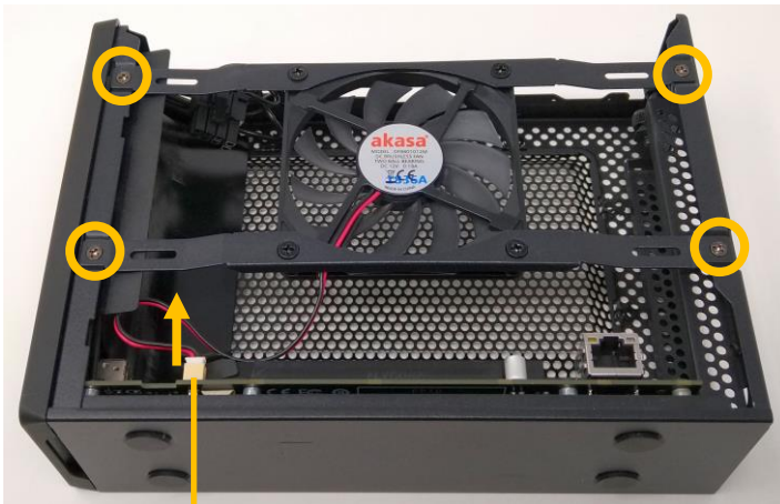
電源コネクタ
